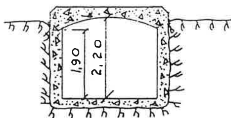
Snitt A-A
