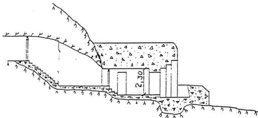
Snitt A-A
