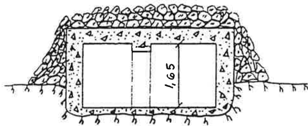
Snitt A-A
