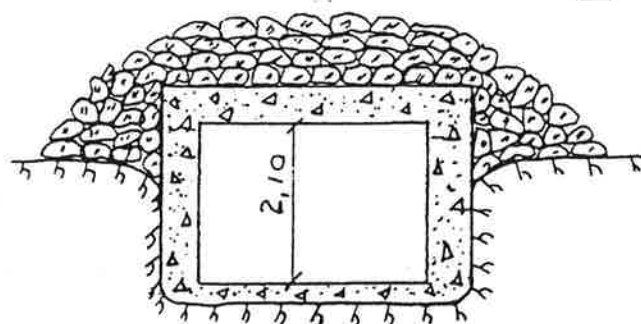
Snitt A-A
