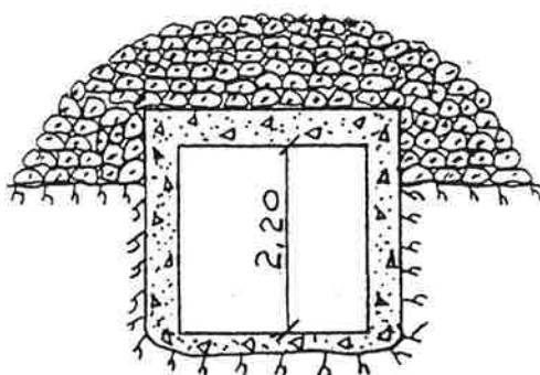
Snitt A-A
