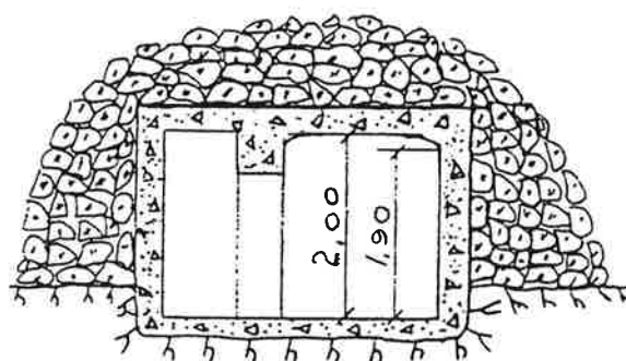
Snitt A-A
