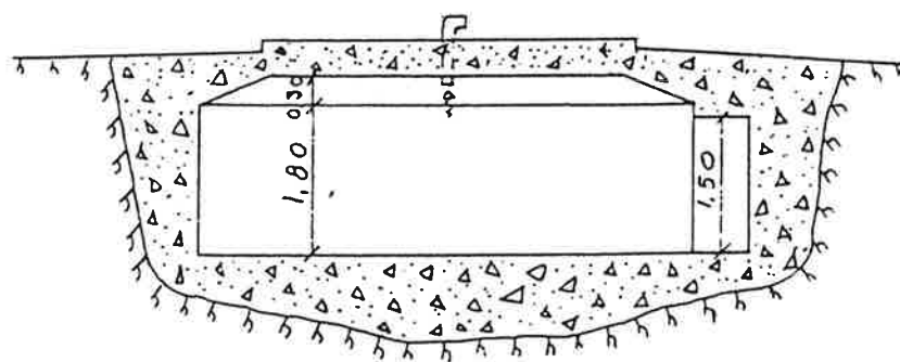
Snitt A-A
