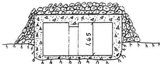
Snitt A-A
