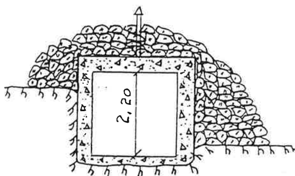
Snitt A-A
