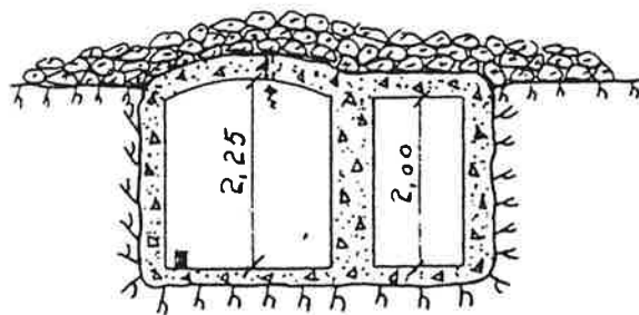
Snitt A-A
