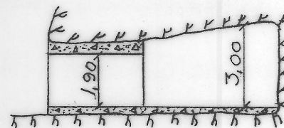
Snitt B-B
