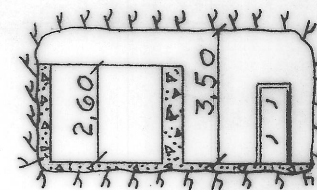
Snitt D-D
